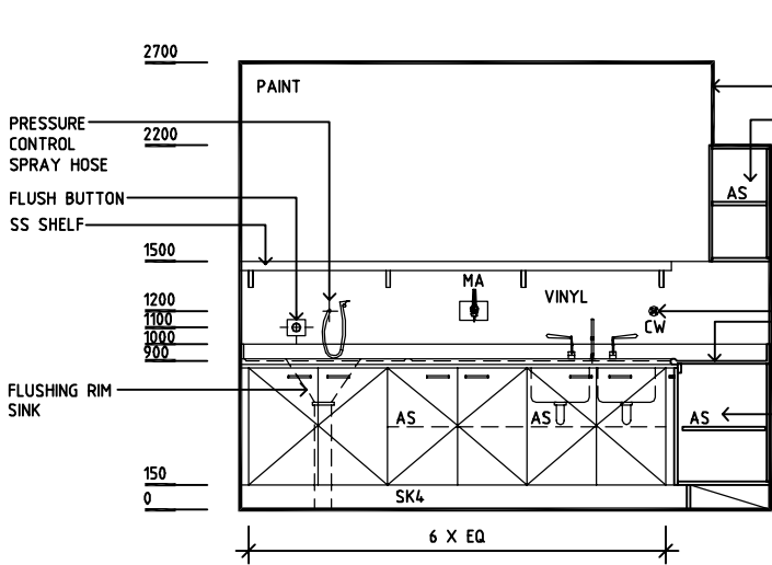
ELEVATION 1
