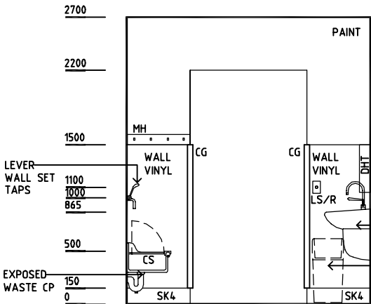
ELEVATION 3
