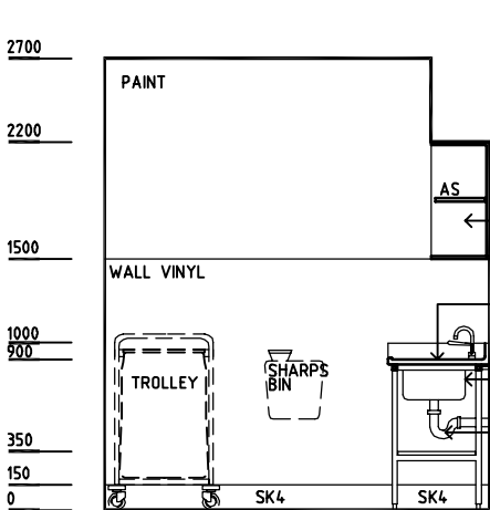
ELEVATION 1
