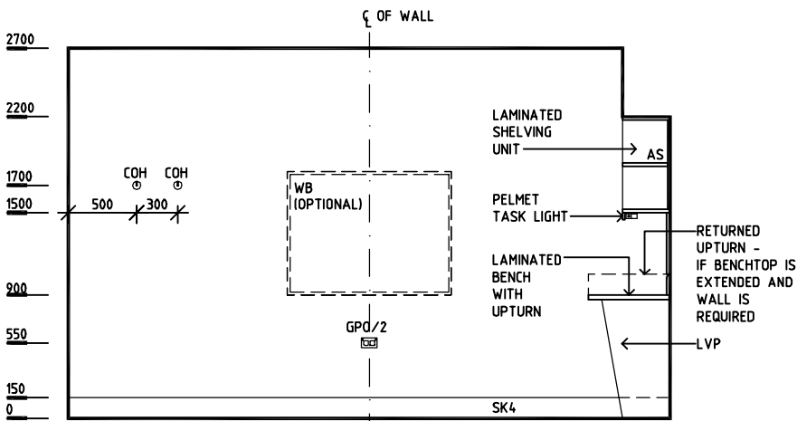
ELEVATION 4
