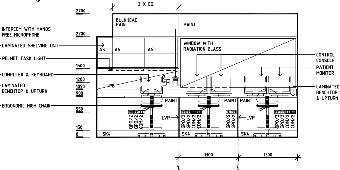
ELEVATION 2
