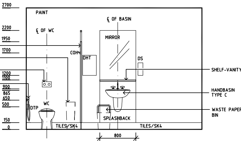
ELEVATION 2
