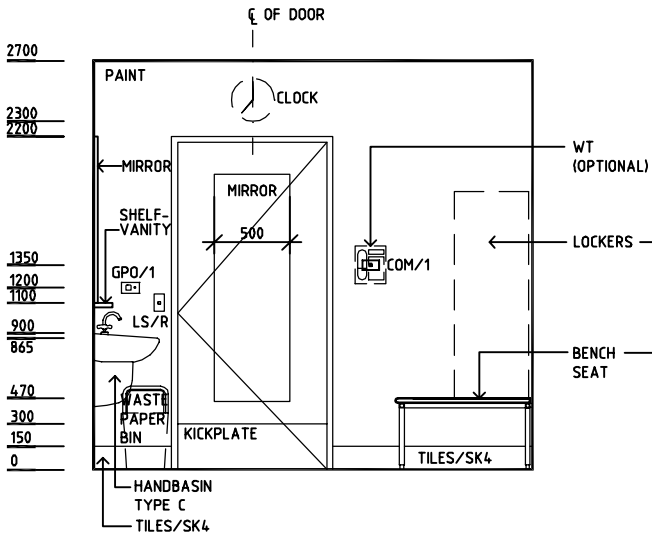
ELEVATION 3
