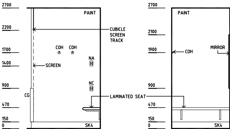
ELEVATION 1
