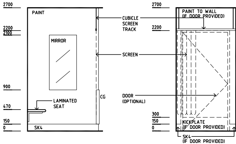
ELEVATION 3
