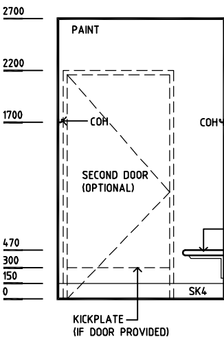
ELEVATION 1
