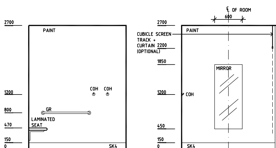
ELEVATION 4
