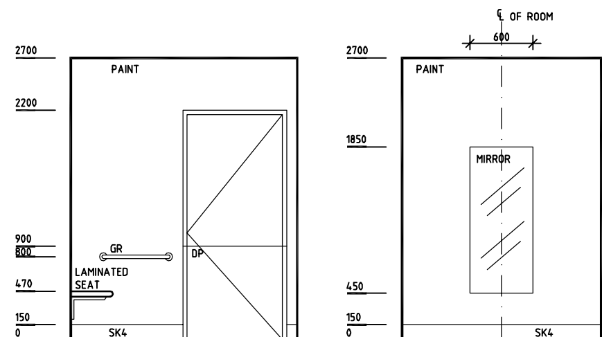
ELEVATION 4
