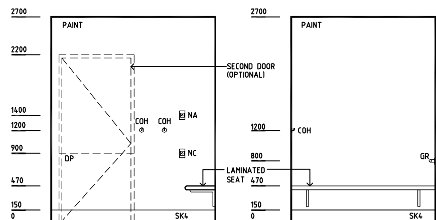
ELEVATION 2
