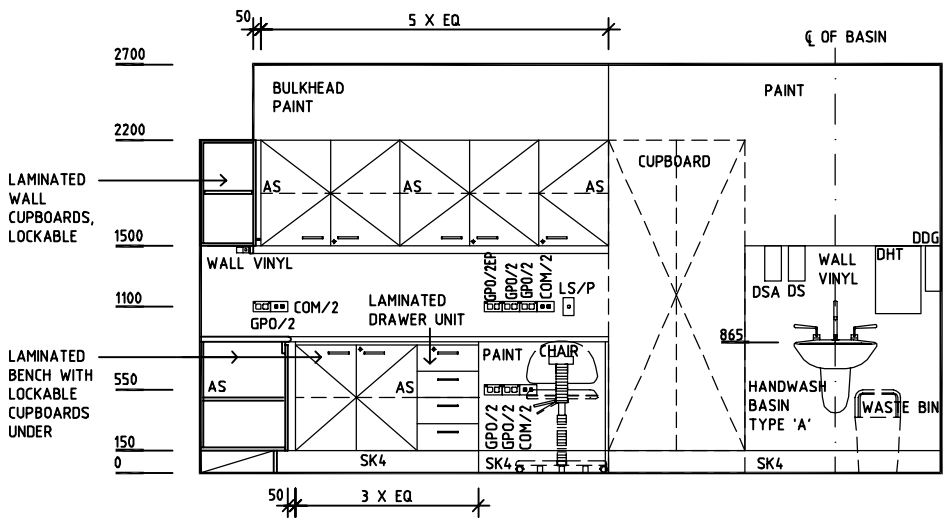
ELEVATION 1
