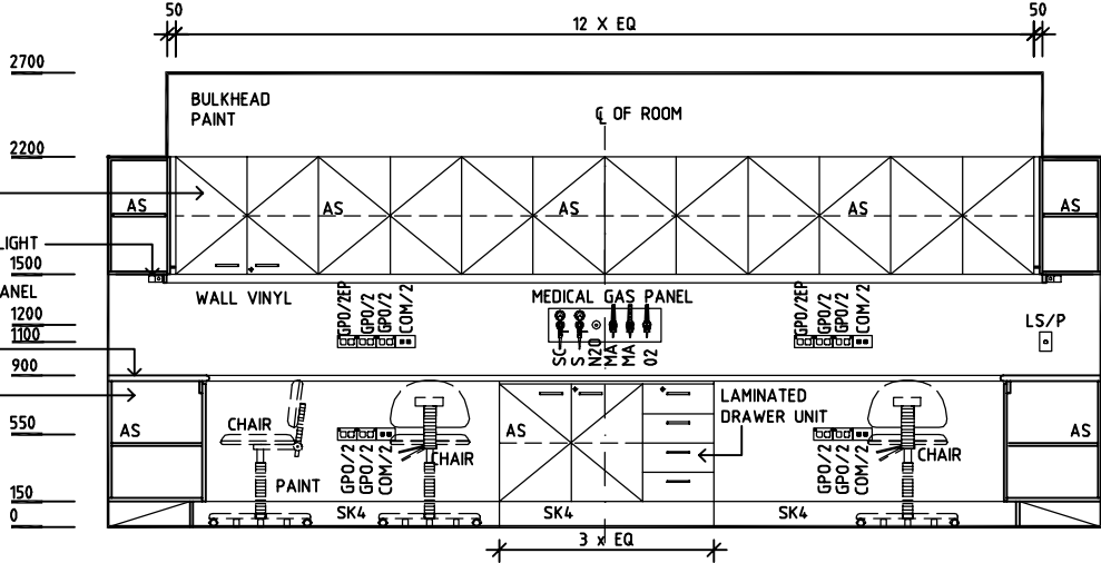
ELEVATION 4
