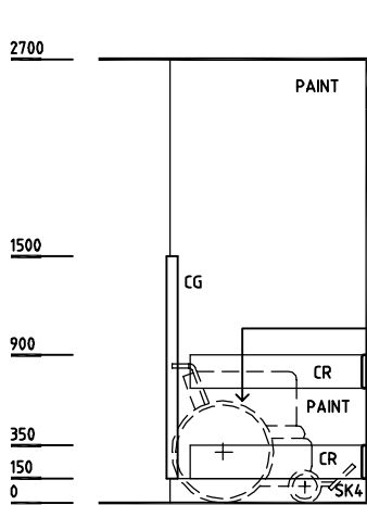
ELEVATION 1
