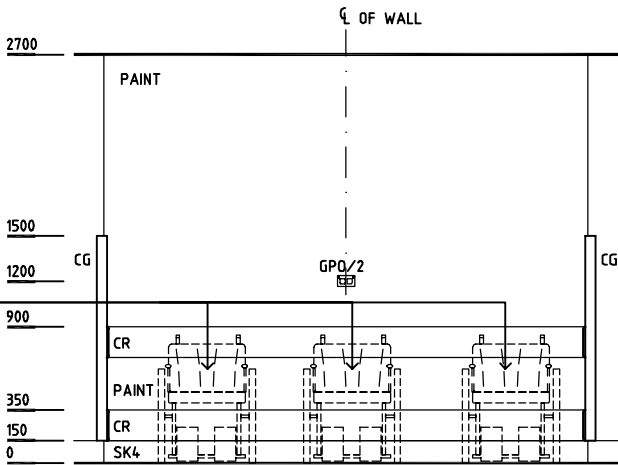
ELEVATION 2
