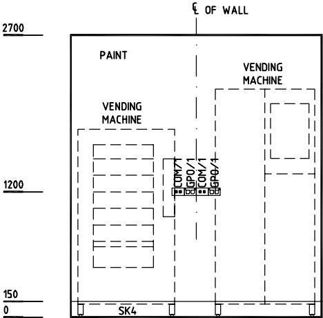
ELEVATION 2
