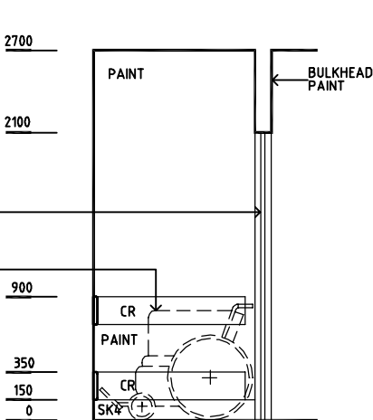
ELEVATION 3
