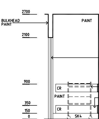
ELEVATION 1
