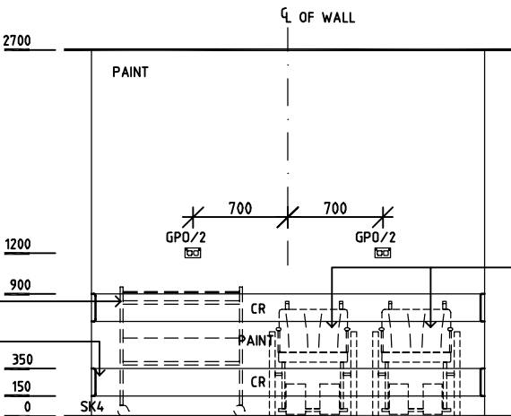
ELEVATION 2
