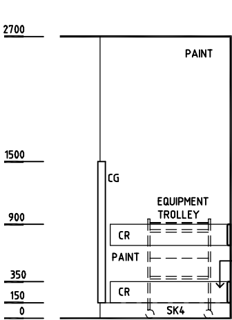
ELEVATION 1
