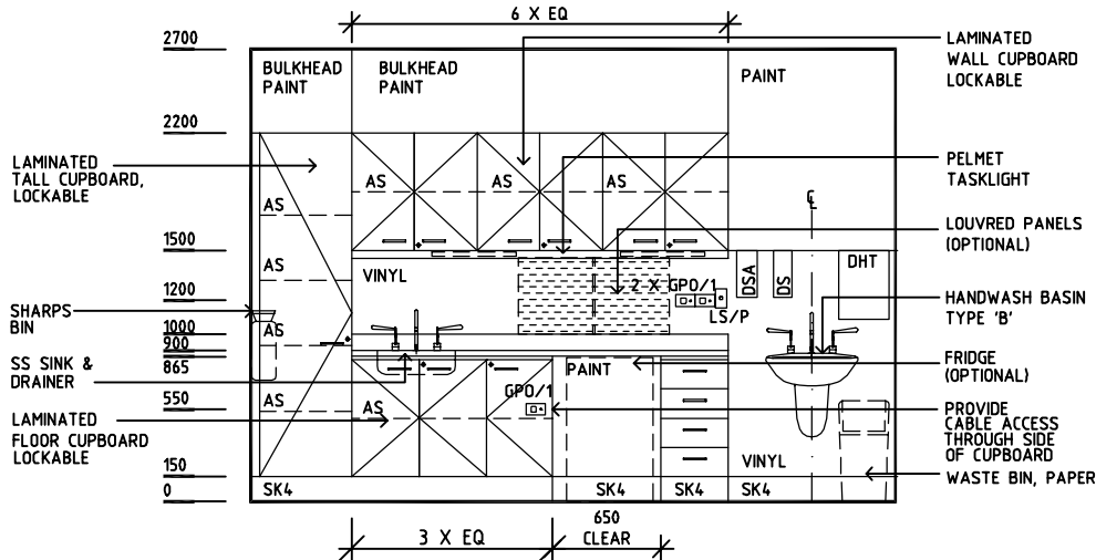
ELEVATION 1
