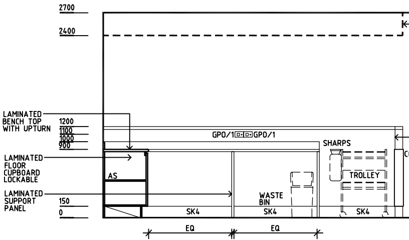
ELEVATION 3
