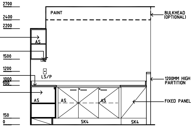
ELEVATION 2
