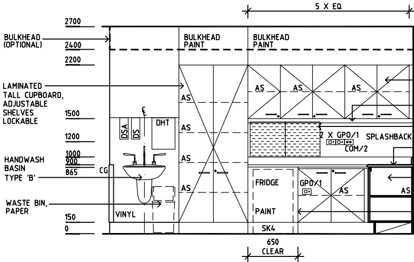
ELEVATION 1
