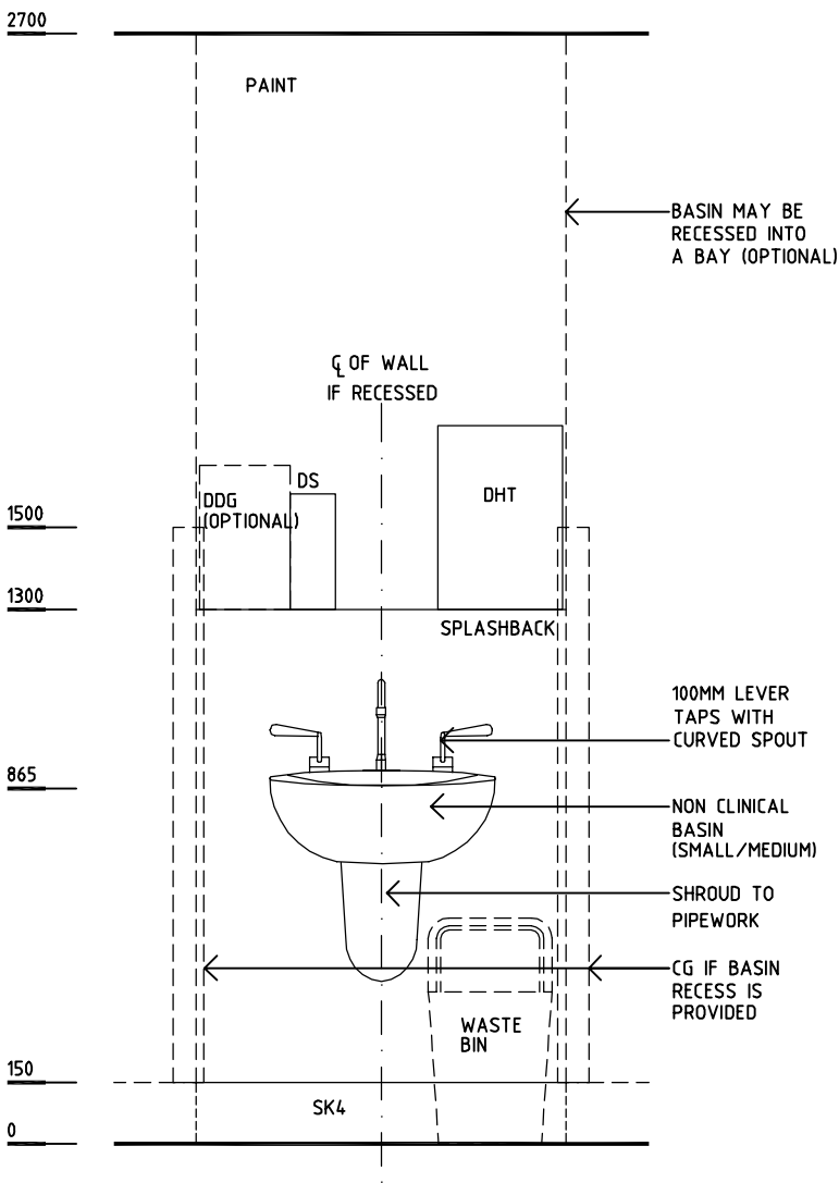
ELEVATION 1
