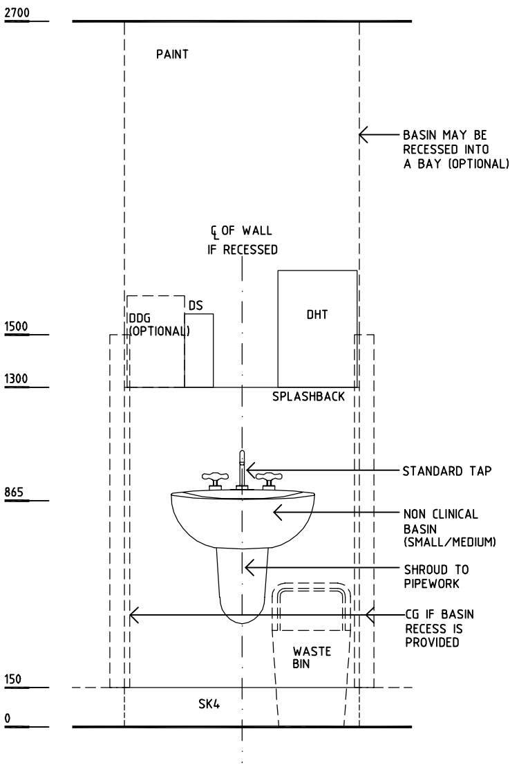
ELEVATION 1
