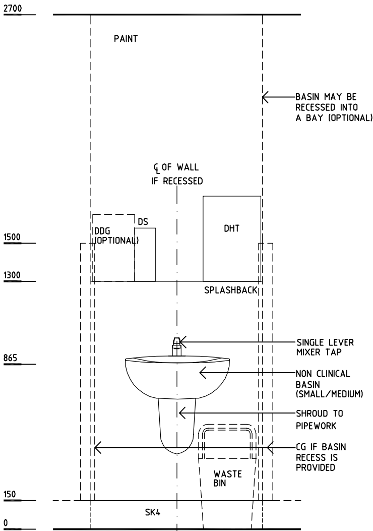
ELEVATION 1
