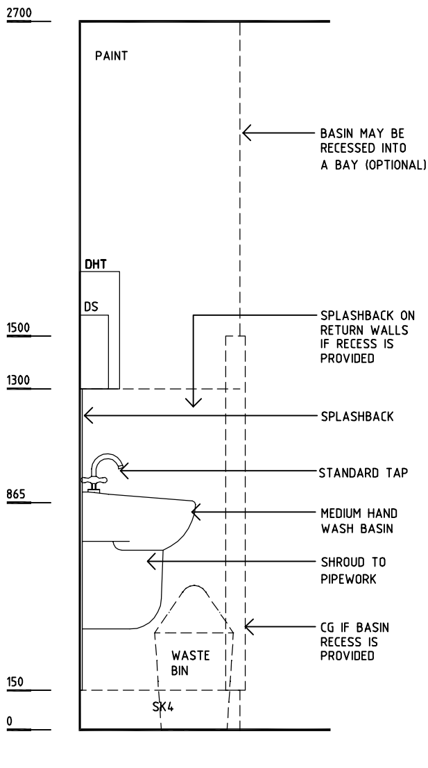
ELEVATION 2
