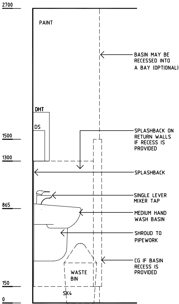
ELEVATION 2
