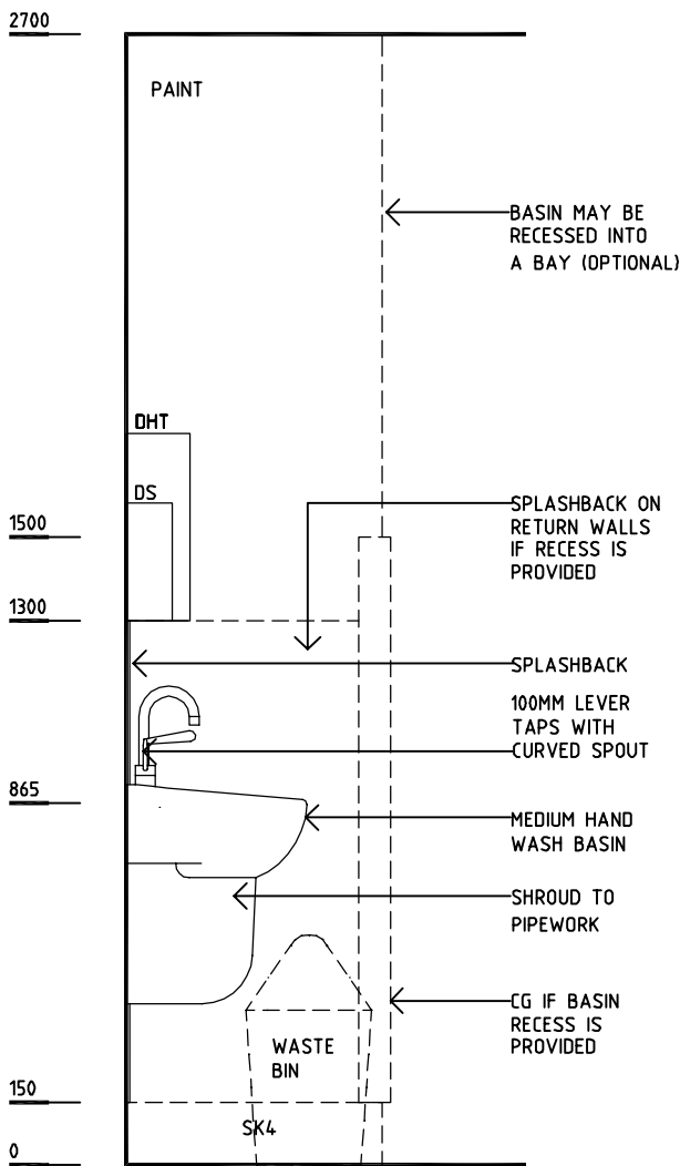
ELEVATION 2
