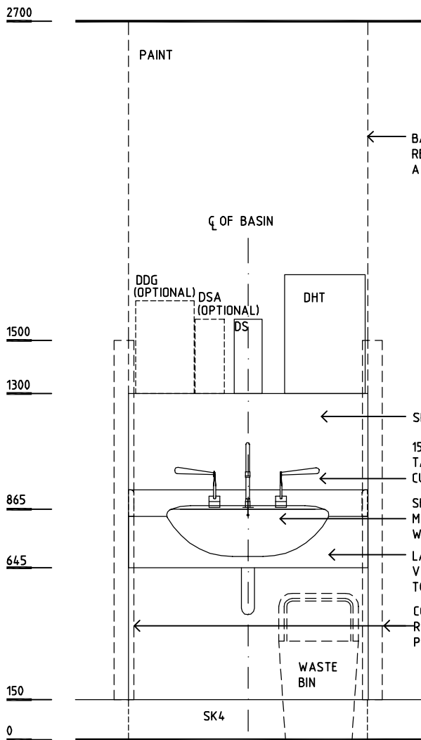
ELEVATION 1
