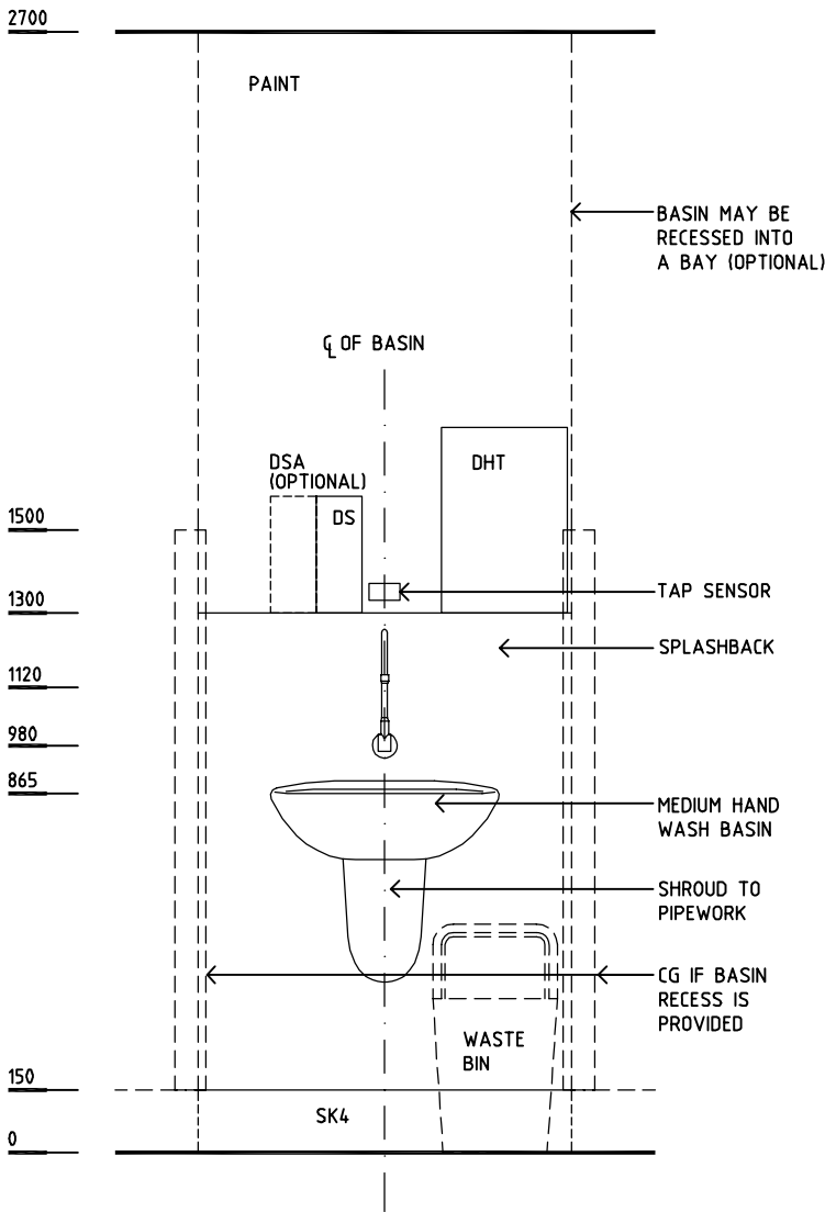
ELEVATION 1
