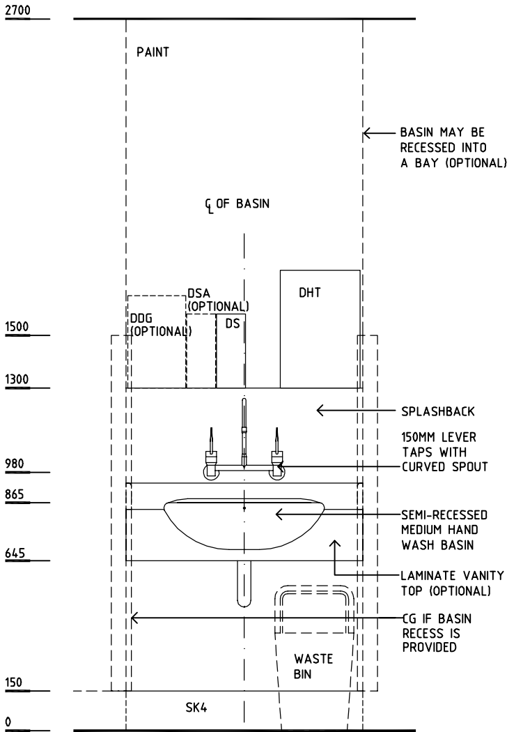
ELEVATION 1
