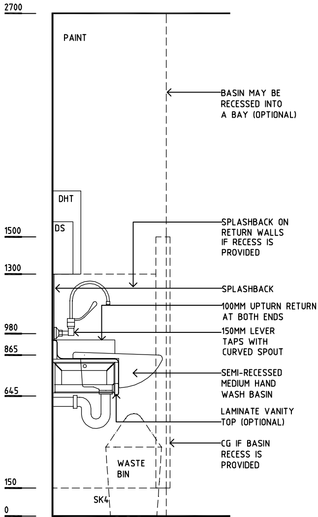
ELEVATION 2
