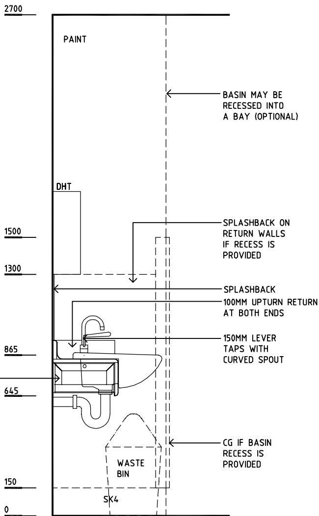
ELEVATION 2
