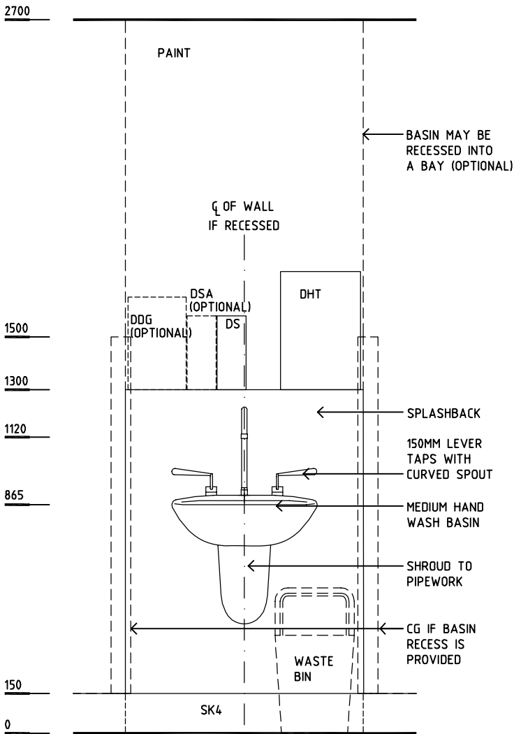
ELEVATION 1
