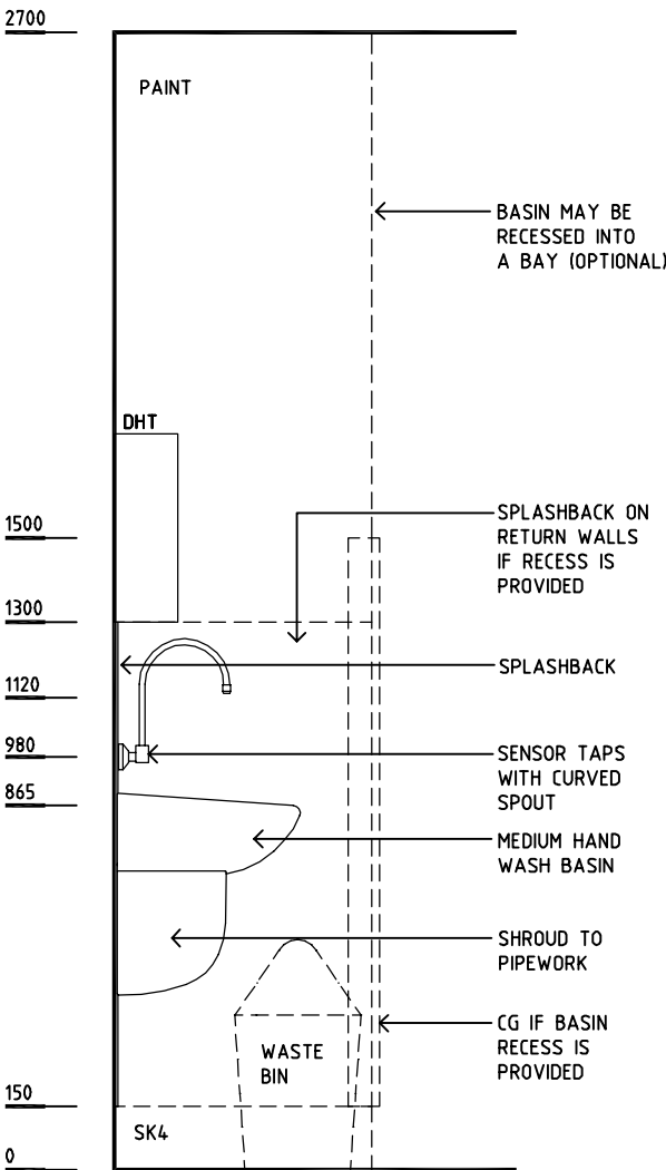
ELEVATION 2
