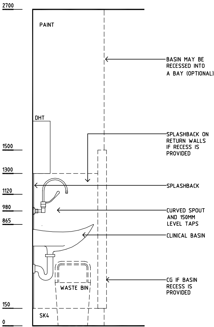
ELEVATION 2
