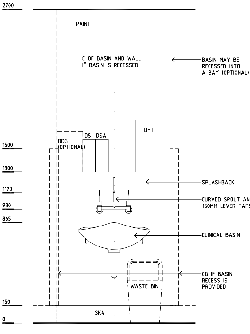
ELEVATION 1
