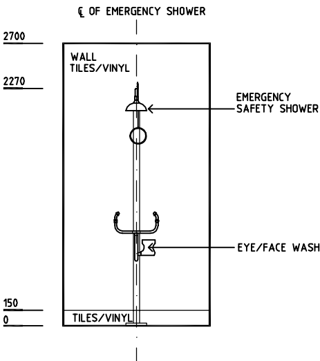
ELEVATION 2
