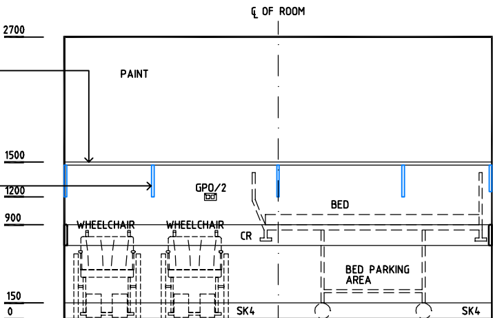
ELEVATION 4
