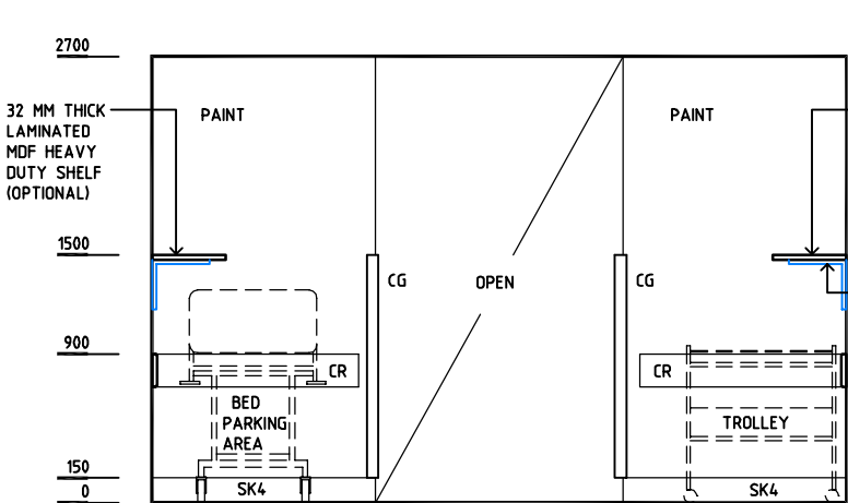
ELEVATION 1
