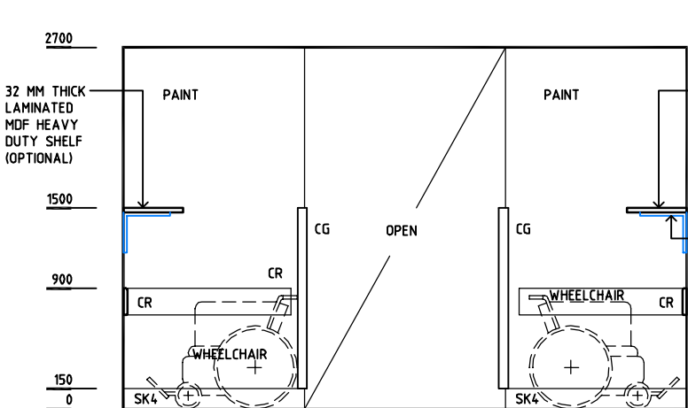
ELEVATION 3
