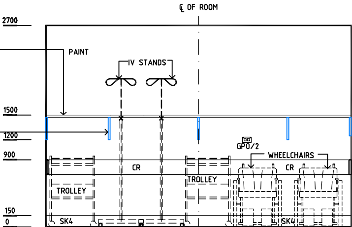
ELEVATION 2
