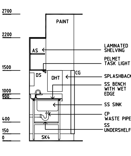
ELEVATION 3
