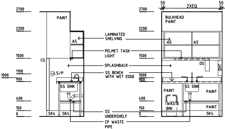
ELEVATION 1
