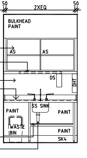
ELEVATION 2
