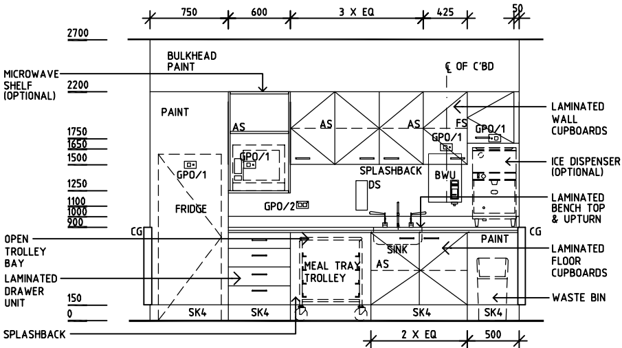
ELEVATION 1
