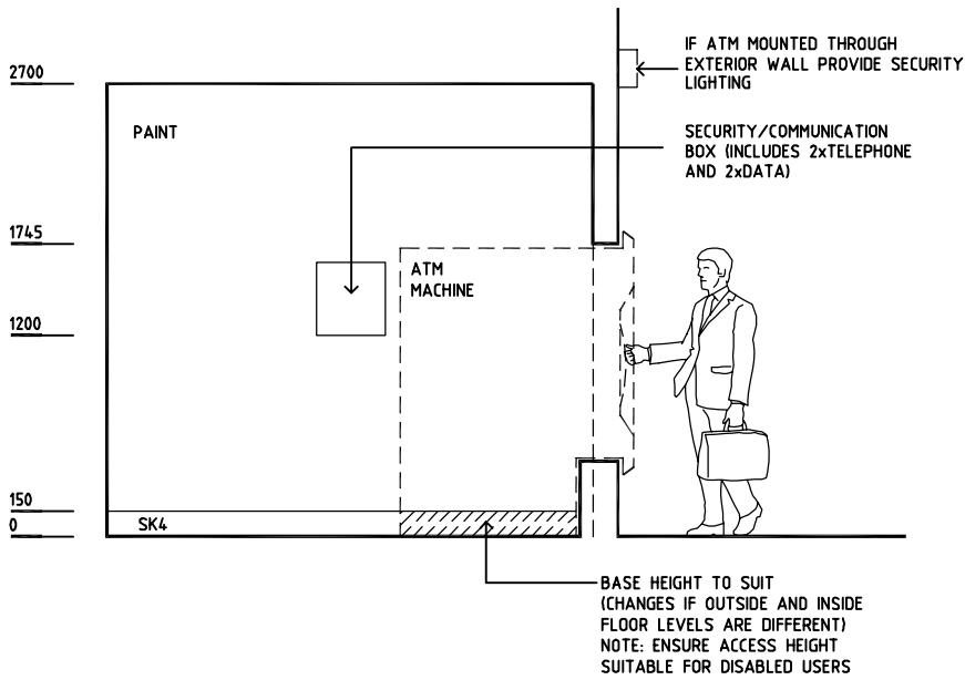
ELEVATION 2
