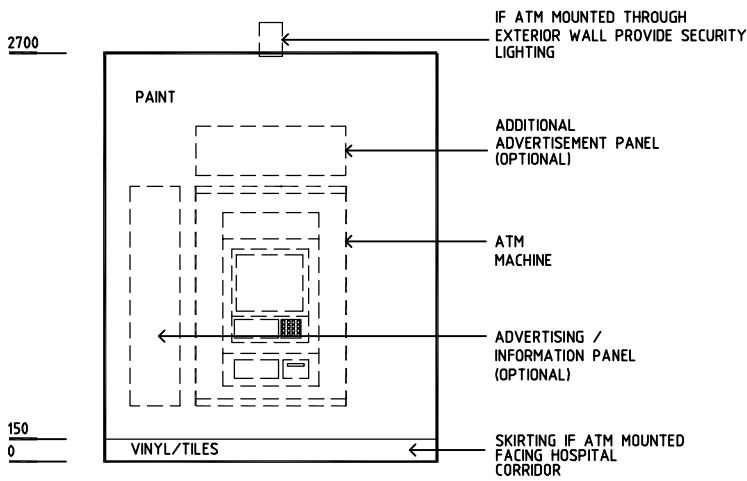
ELEVATION 3
