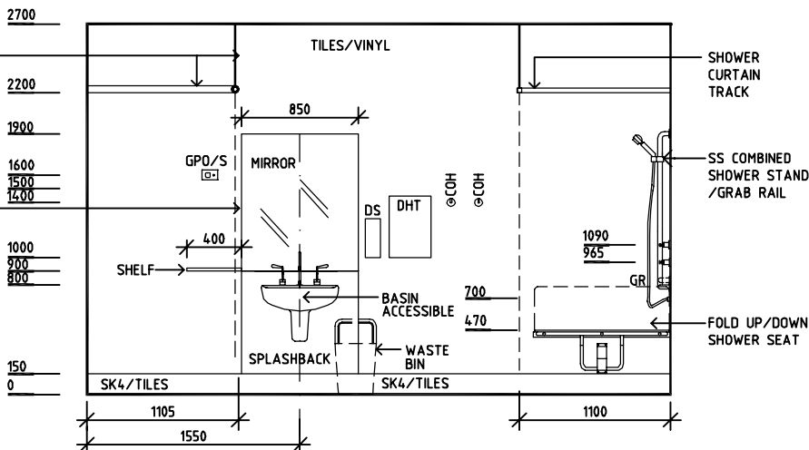
ELEVATION 2
