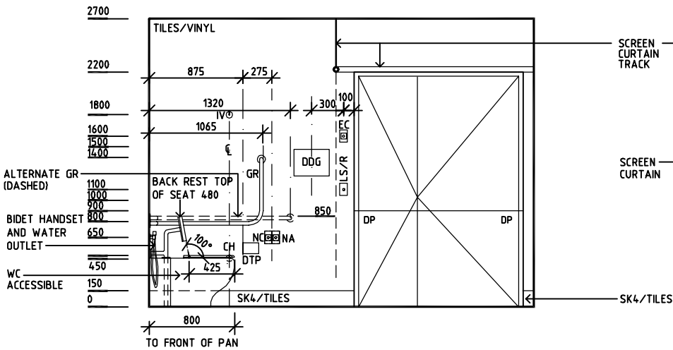
ELEVATION 1
