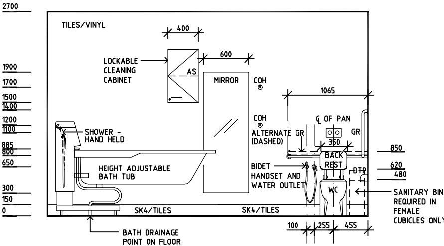
ELEVATION 4
