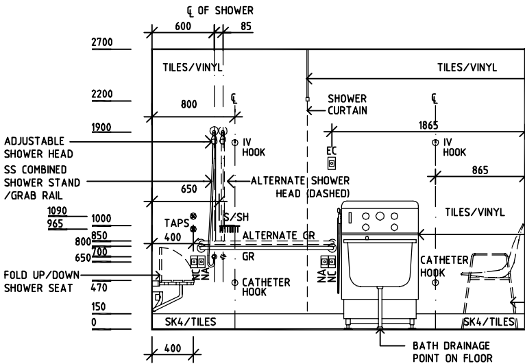
ELEVATION 3
