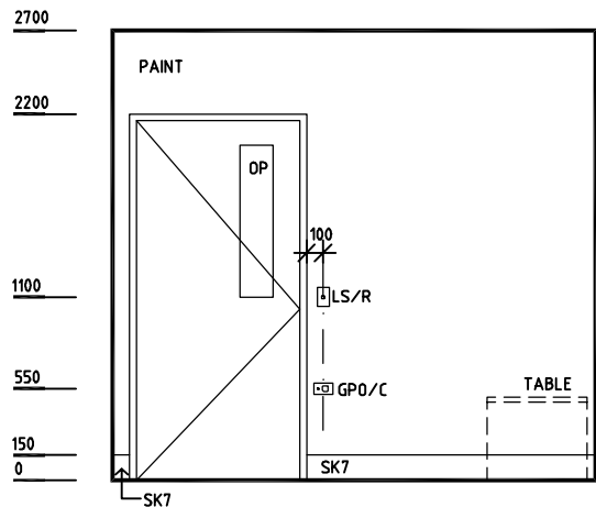
ELEVATION 3
