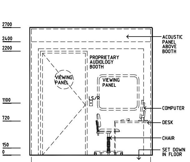
ELEVATION 1
