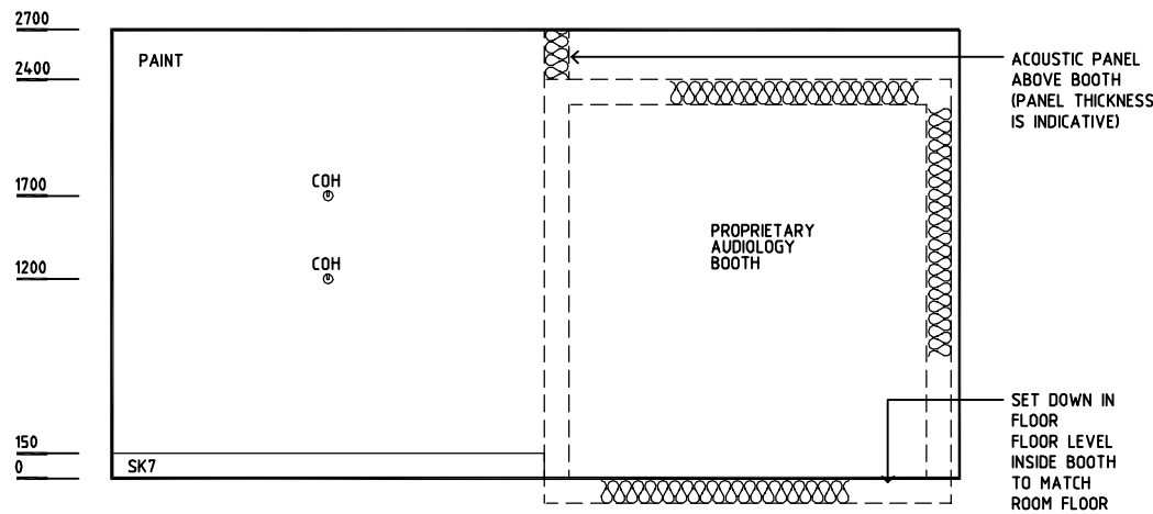
ELEVATION 4
