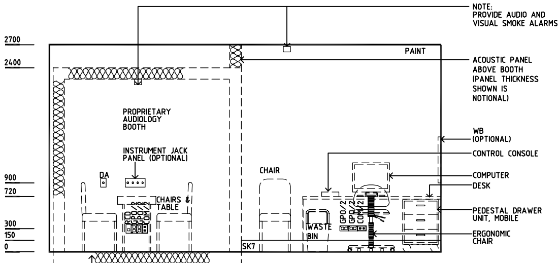
ELEVATION 2
