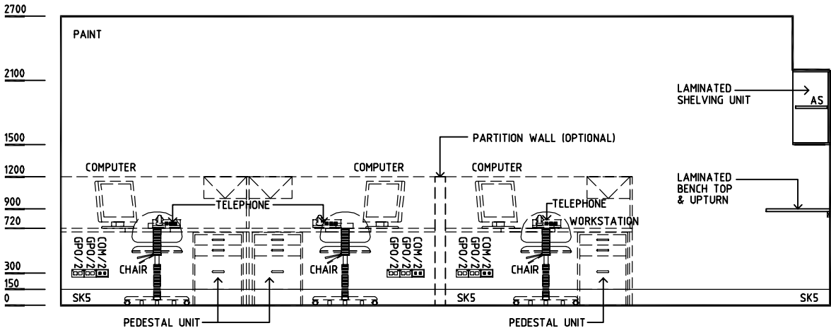
ELEVATION 2
