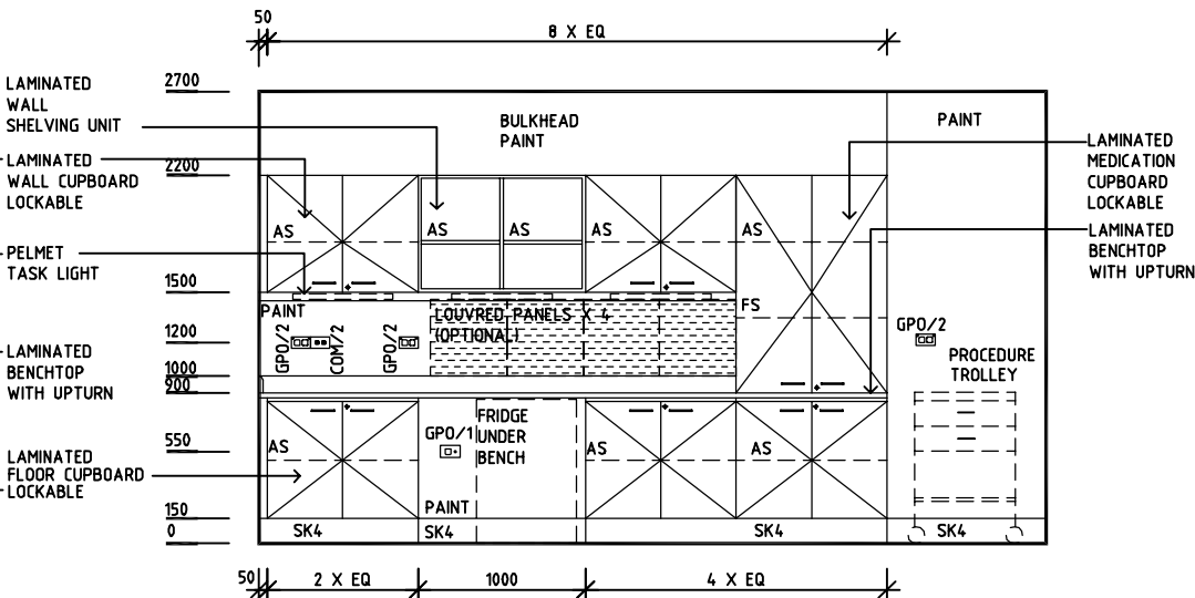
ELEVATION 2
