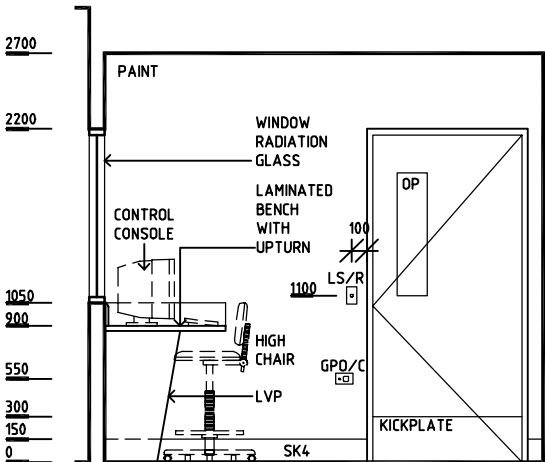
ELEVATION 3
