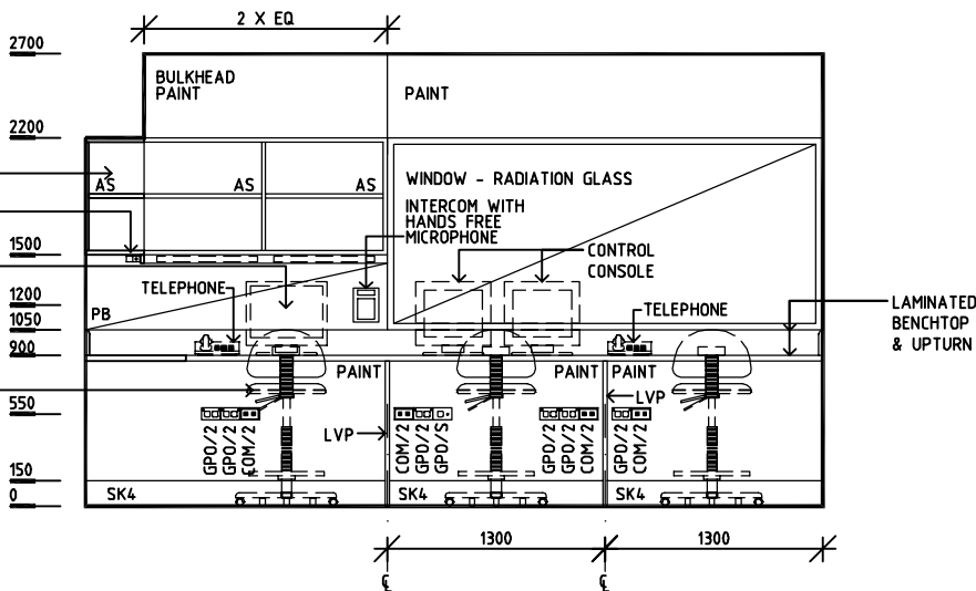
ELEVATION 2
