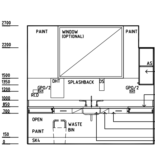
ELEVATION 1
