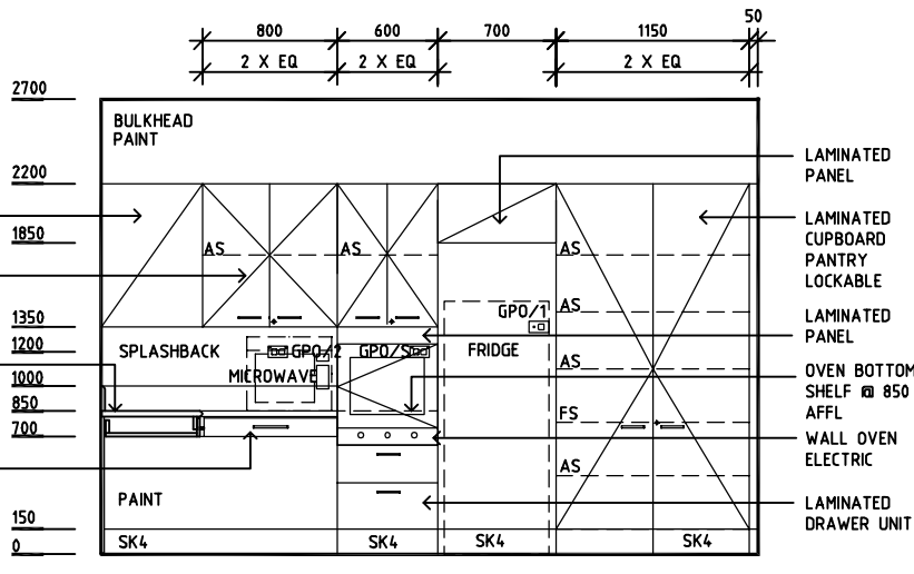
ELEVATION 2
