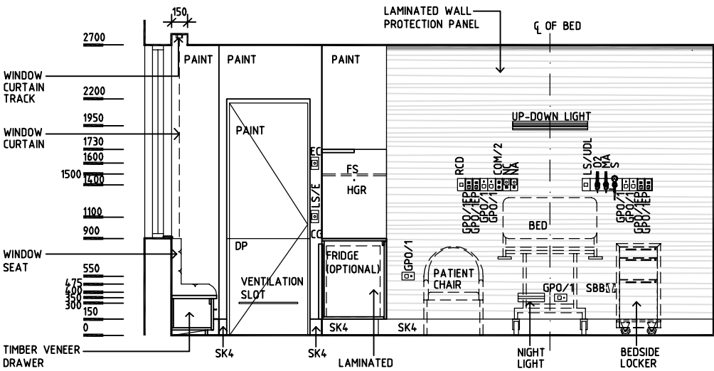
ELEVATION 2
