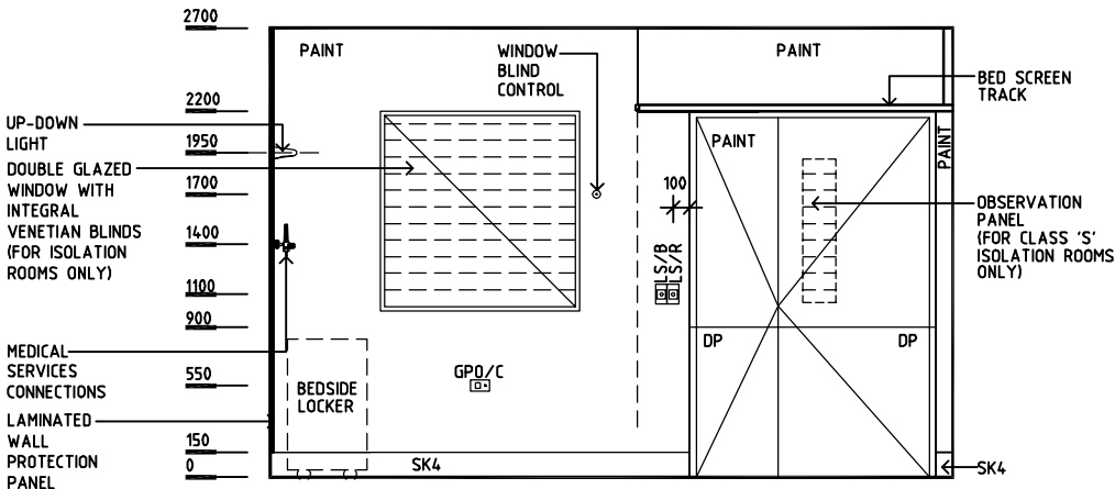
ELEVATION 3
