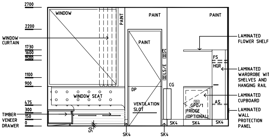
ELEVATION 1
