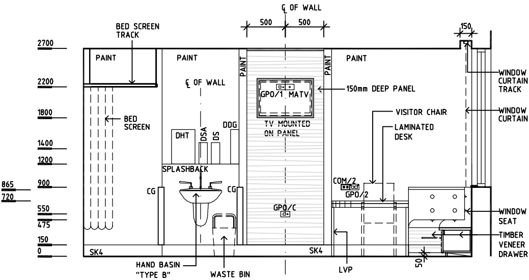
ELEVATION 4
