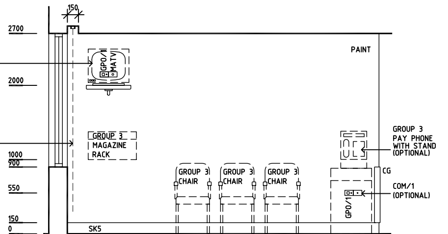
ELEVATION 2
