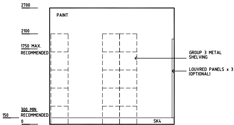
ELEVATION 1
