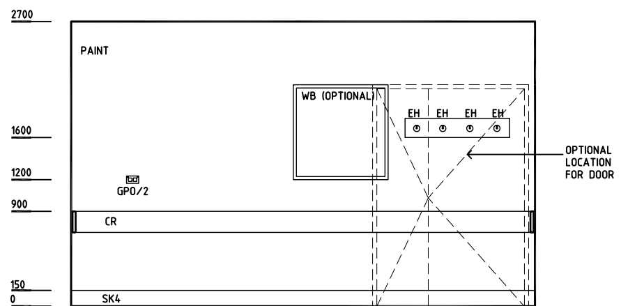
ELEVATION 2
