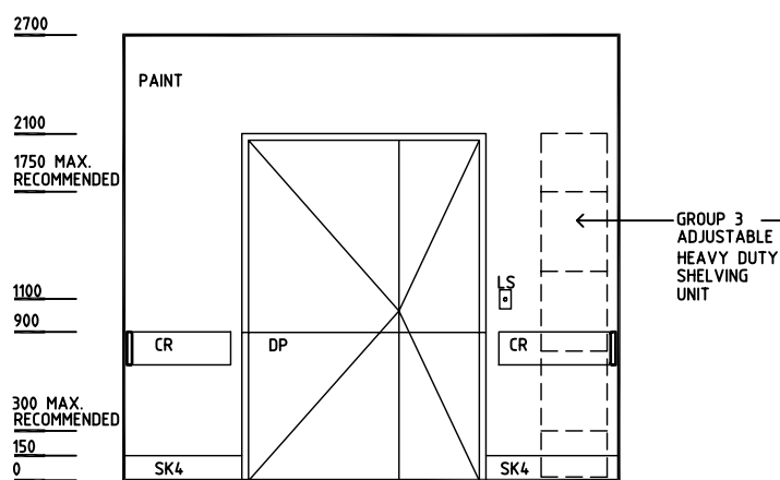
ELEVATION 3
