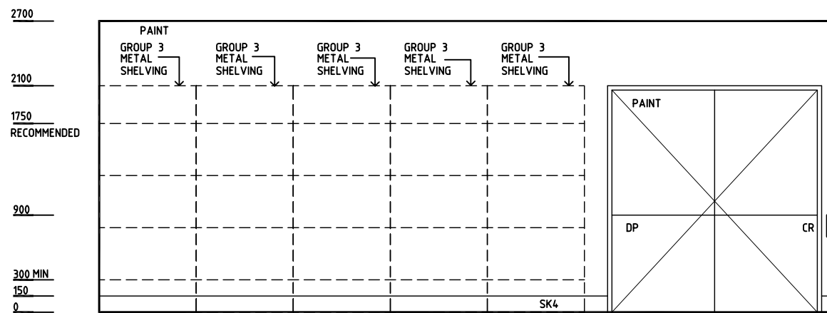
ELEVATION 1
