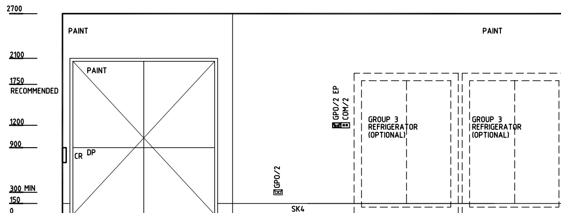
ELEVATION 3
