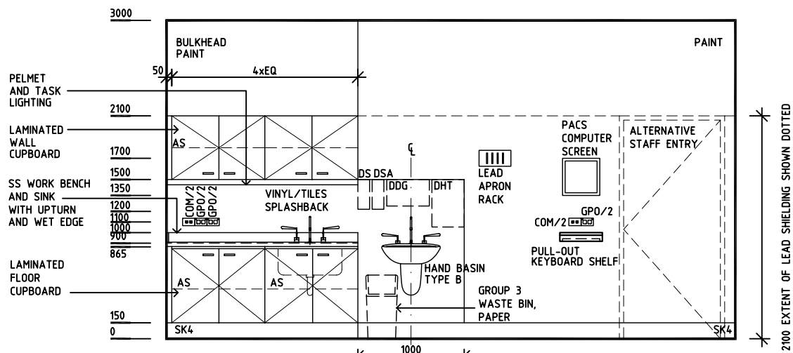
ELEVATION 4
