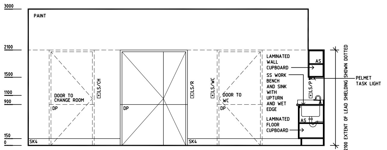
ELEVATION 3
