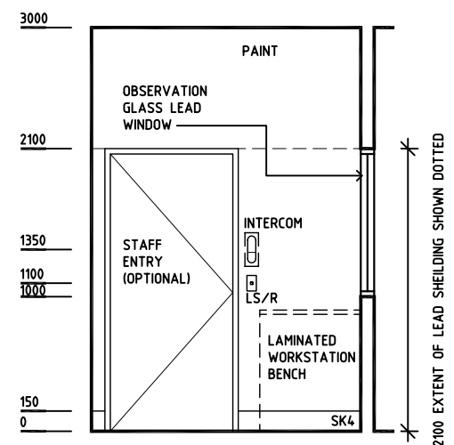
ELEVATION 6
