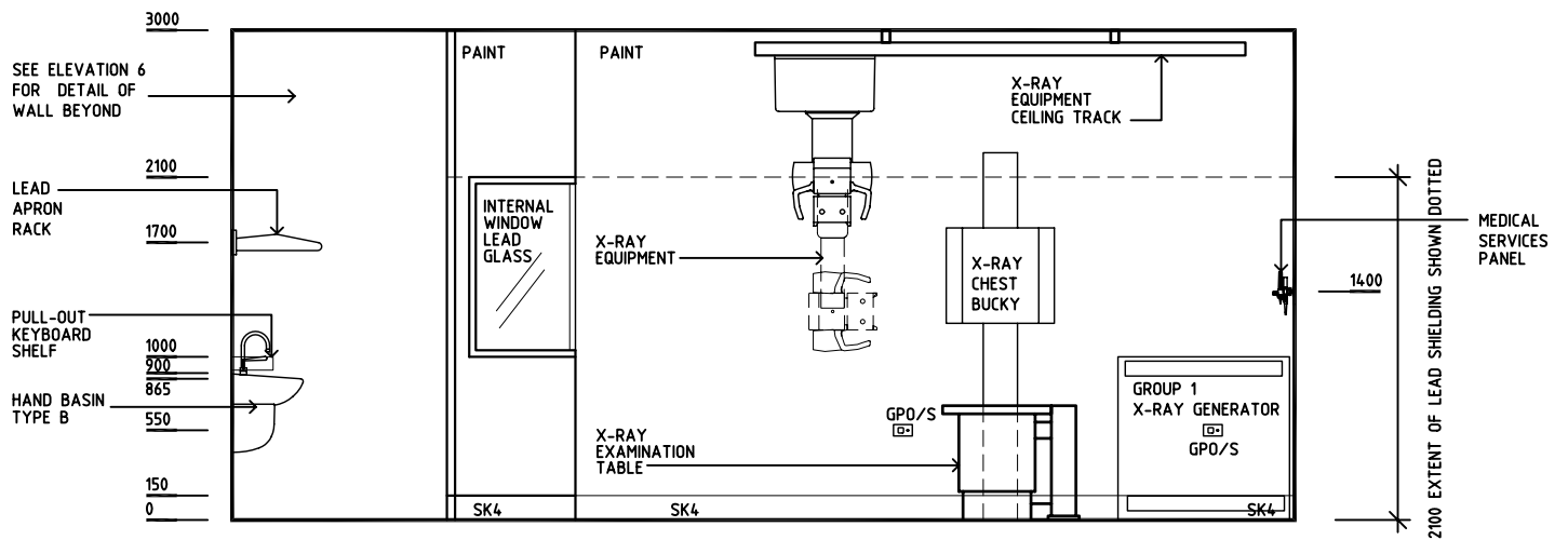
ELEVATION 1
