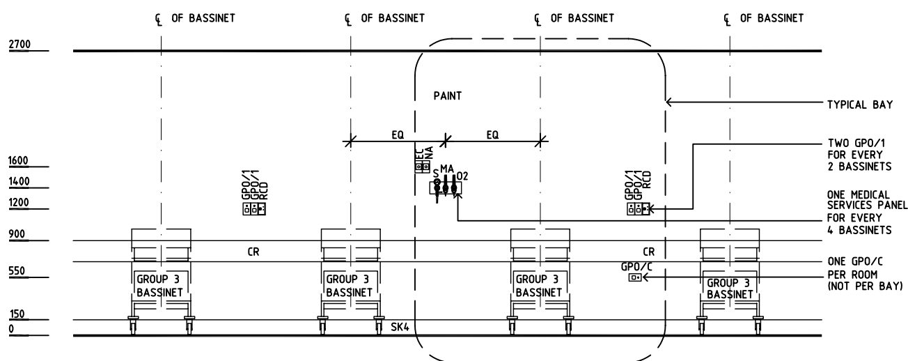
ELEVATION 1
