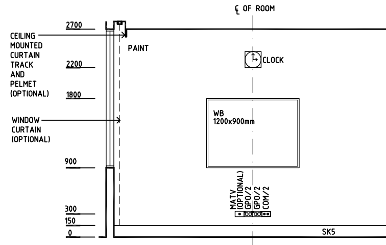
ELEVATION 2
