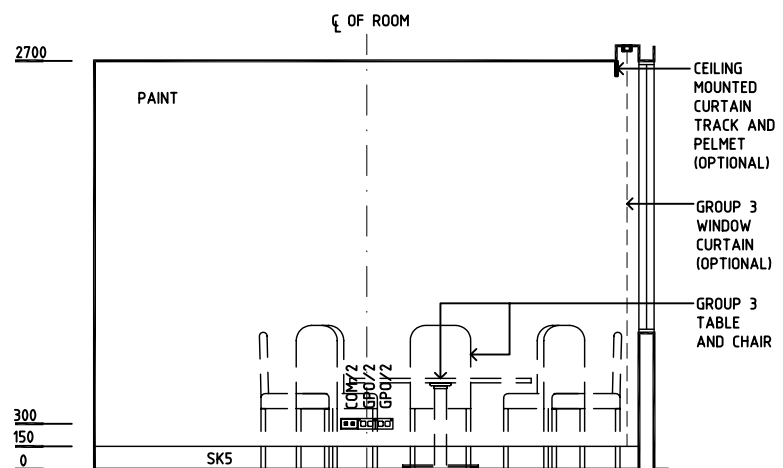
ELEVATION 4
