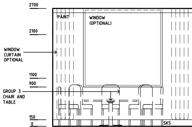
ELEVATION 1
