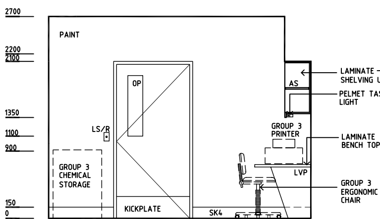
ELEVATION 3
