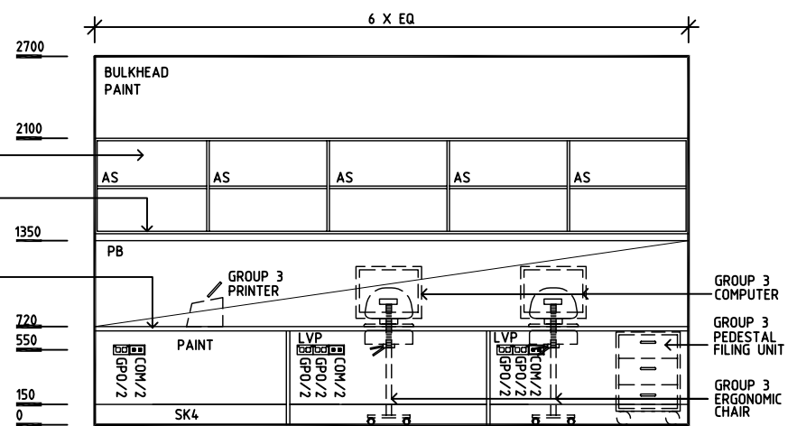
ELEVATION 4
