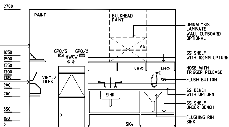
ELEVATION 2
