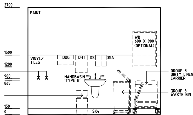
ELEVATION 4
