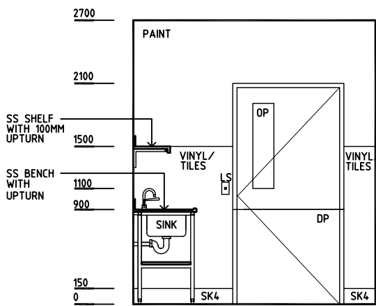
ELEVATION 3
