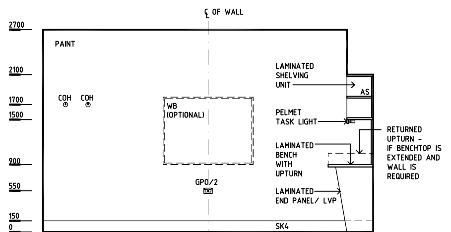
ELEVATION 4
