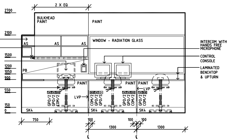
ELEVATION 2
