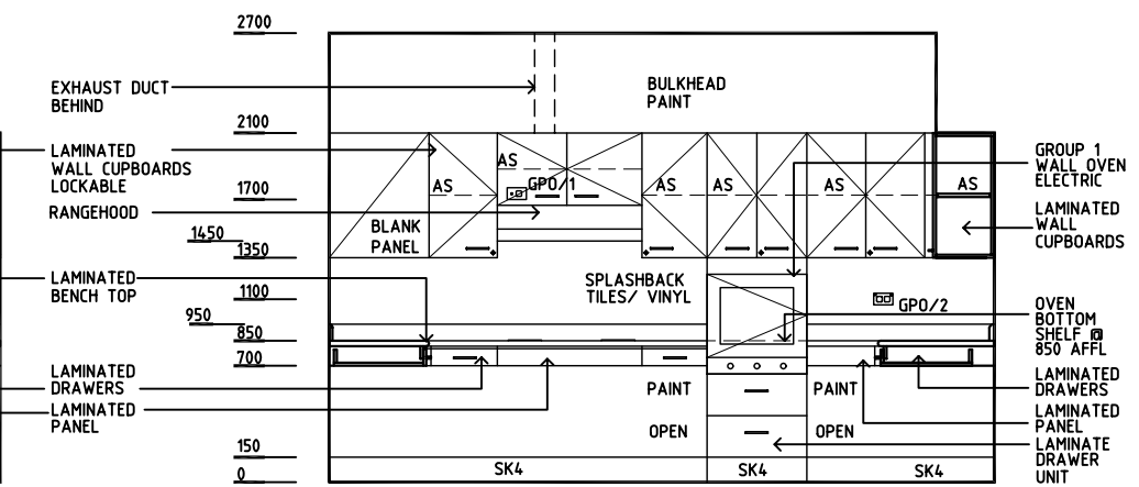
ELEVATION 2
