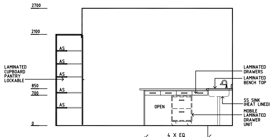
ELEVATION 4
