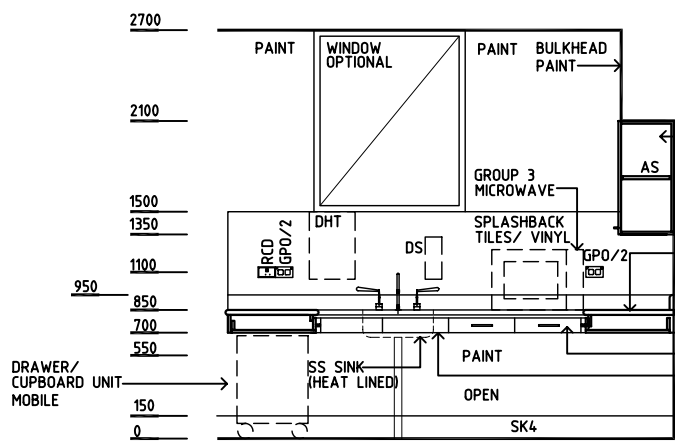
ELEVATION 1
