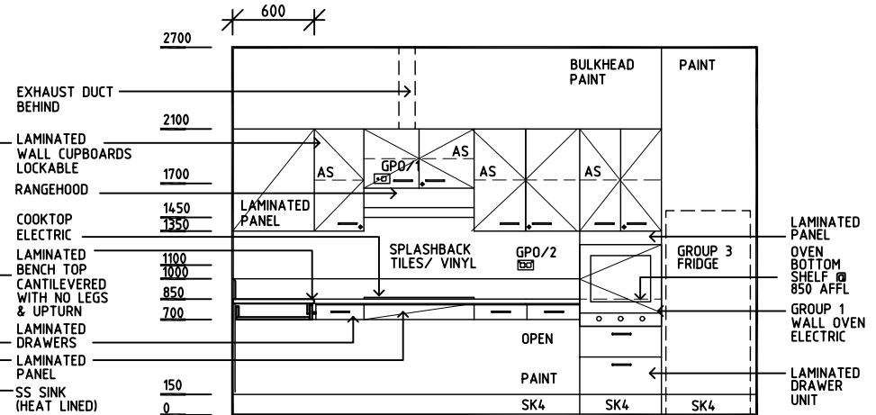
ELEVATION 2
