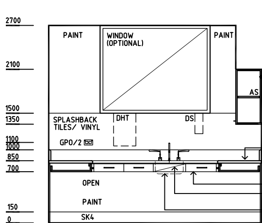
ELEVATION 1
