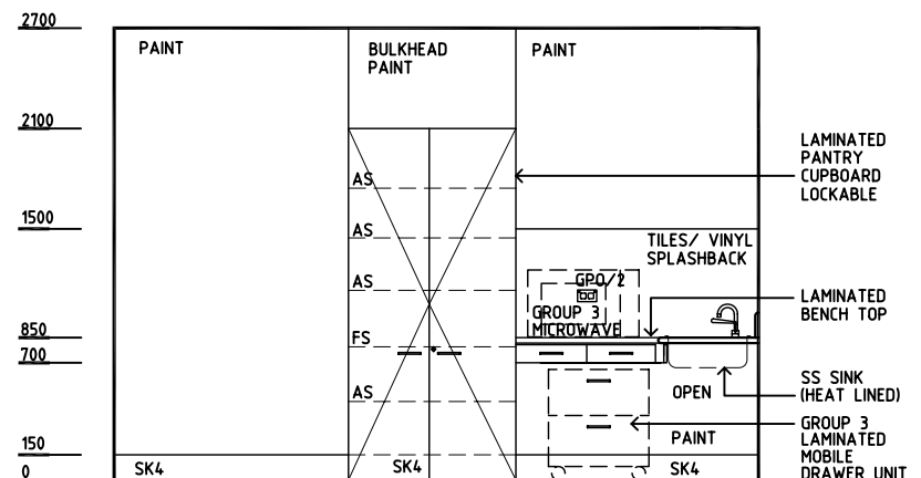
ELEVATION 4
