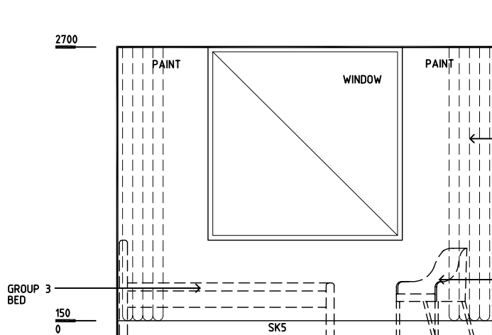
ELEVATION 1
