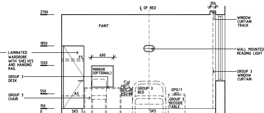
ELEVATION 4
