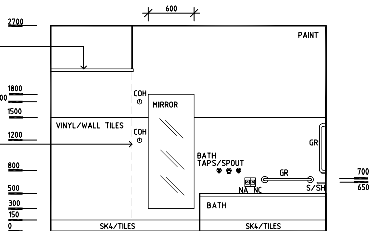
ELEVATION 4
