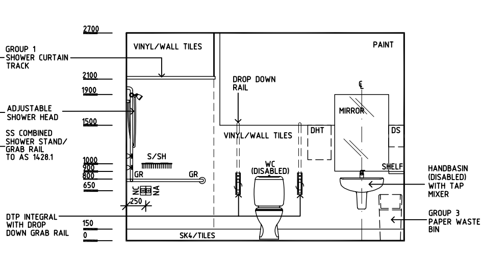
ELEVATION 2
