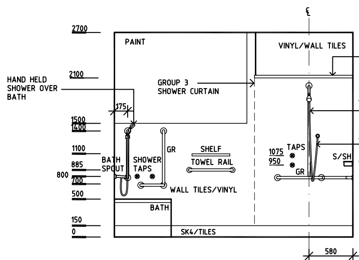
ELEVATION 1
