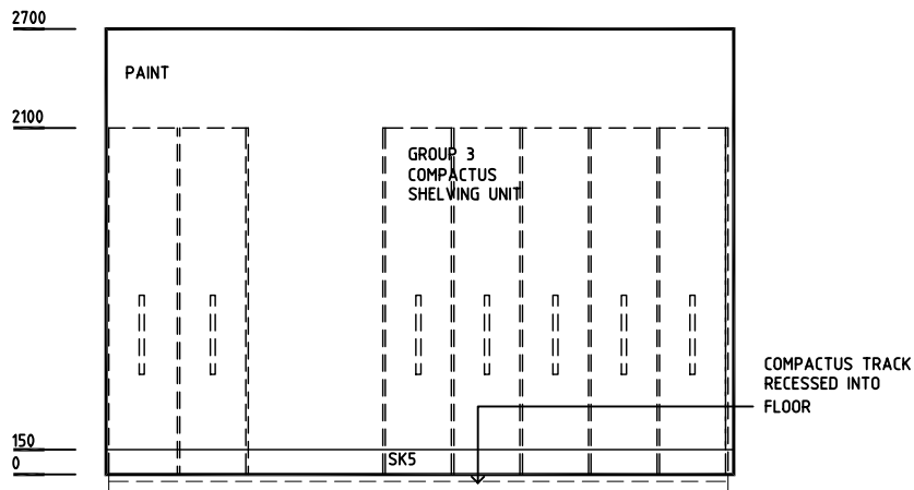
ELEVATION 1
