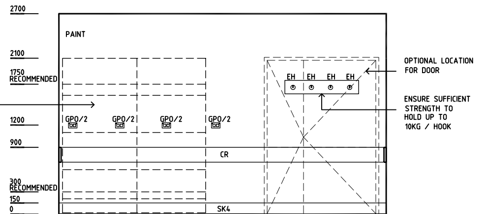
ELEVATION 2
