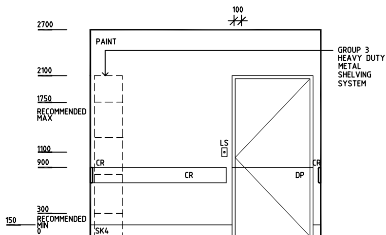
ELEVATION 3
