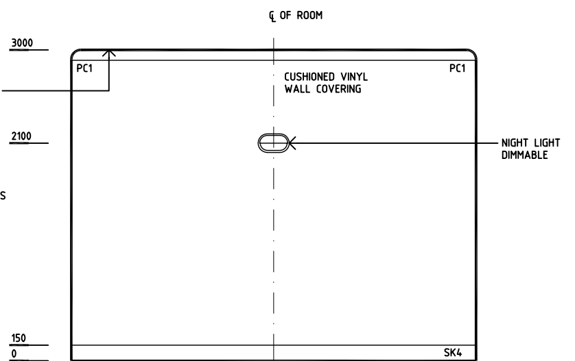
ELEVATION 2
