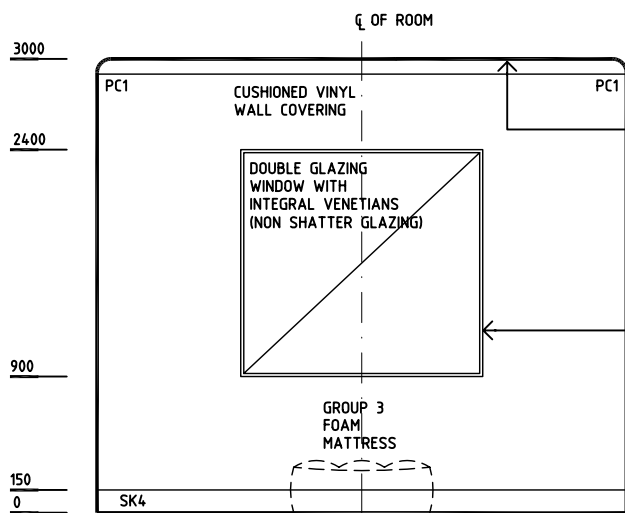
ELEVATION 1
