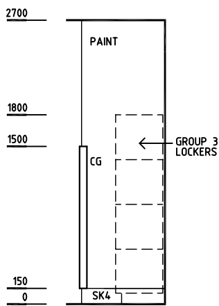
ELEVATION 1
