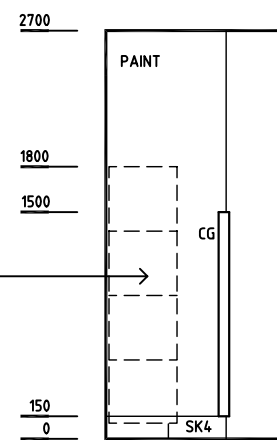
ELEVATION 3
