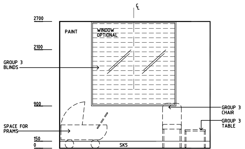
ELEVATION 1
