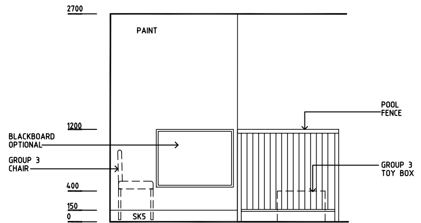
ELEVATION 2
