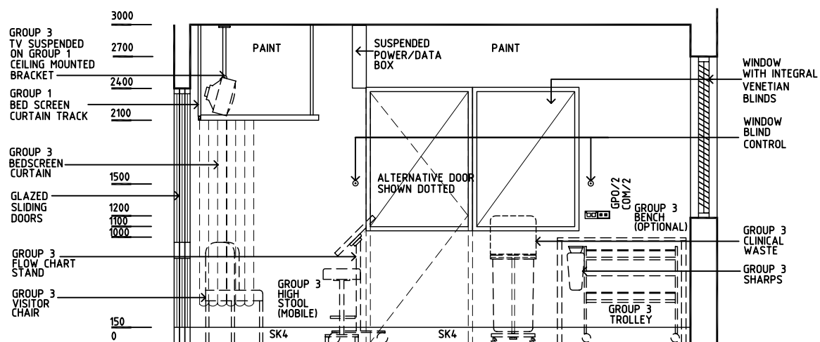
ELEVATION 3
